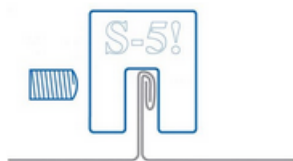
Montage B-Klemme auf Kupfer-Doppelstehfalz
