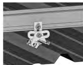
Montage von Schienen mit seitlichem Schraubkanal
