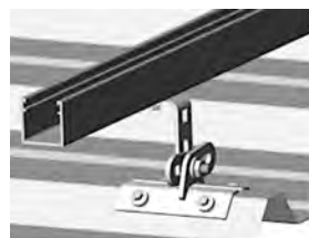
Montage von Schienen mit unten liegendem Schraubkanal
