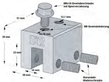
S-5!® S-Klemme
