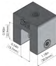
S-5!® S-Mini
