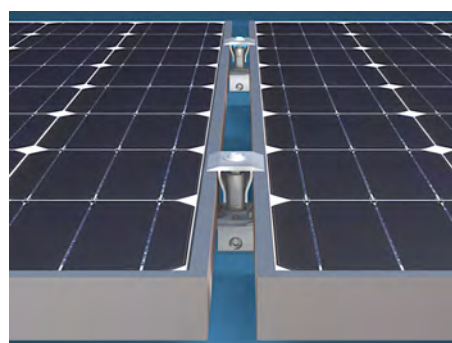
Dachparallele Montage quer zum Falz mit dem PV-Kit 2.0 MidGrab und E-Mini auf Doppelstehfalzdach: universell als End- und Mittel-Klemme einsetzbar.
