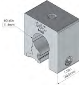
S-5!® Z-Mini
