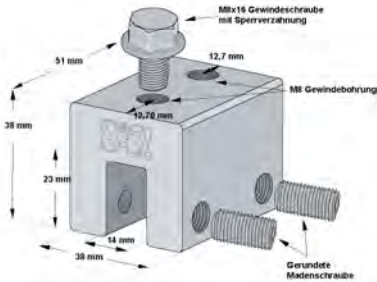
S-5!® S-Klemme
