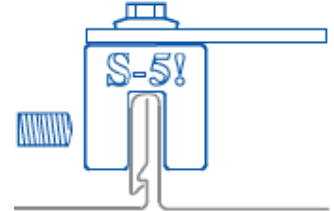
S-Klemme / S-Mini mit Adapterblech
